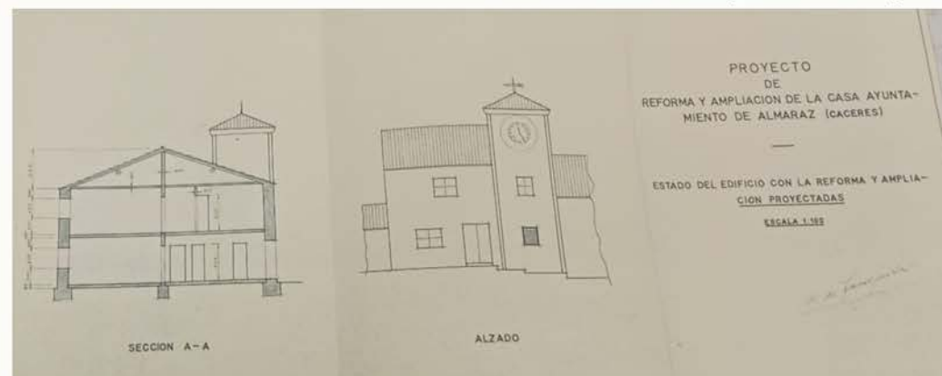
1962. Almaraz Proyecto de la reforma y ampliación de la Casa Ayuntamiento de Almaraz. Plano del estado del edificio con la reforma y ampliación proyectadas, escala 1:100. Varios tamaños, papel. Ayuntamiento de Almaraz ES.10019. AMUALM/03.01.06
