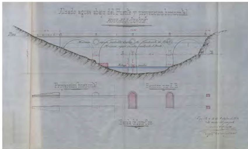
1892. Proyecto de obra sobre río Almonte.
