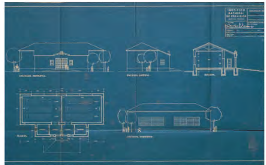
1927, junio, 10. Madrid Planos del edificio destinado a Escuelas Nacionales. 5 hojas, varios tamaños, papel. Ayuntamiento de Portezuelo ES.10513. AMUPTZ/03.01.06/00146/003
